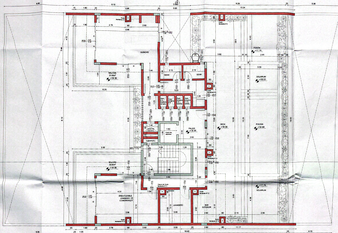
PLANTA DE TERRAZA ESCALA 1:50
