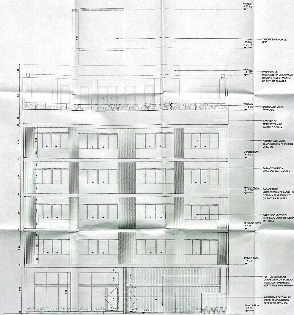
FACHADA FRONTAL ESCALA 1:50
