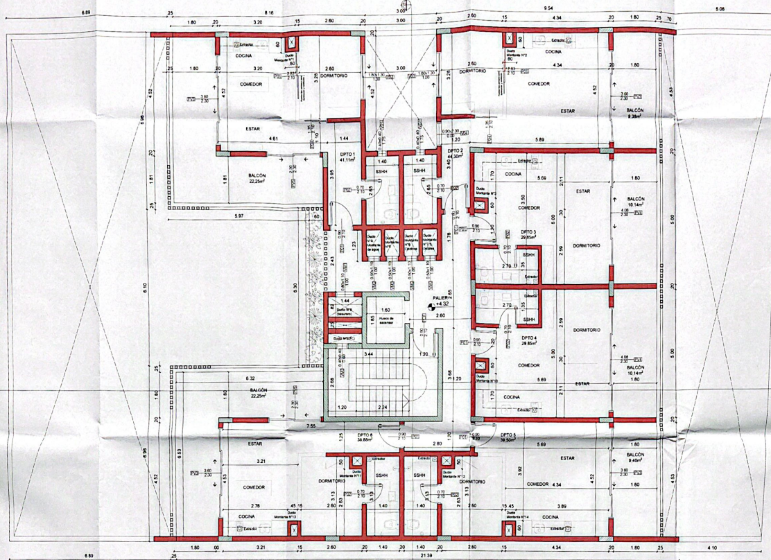
PLANTA TIPO ESCALA 1:50
